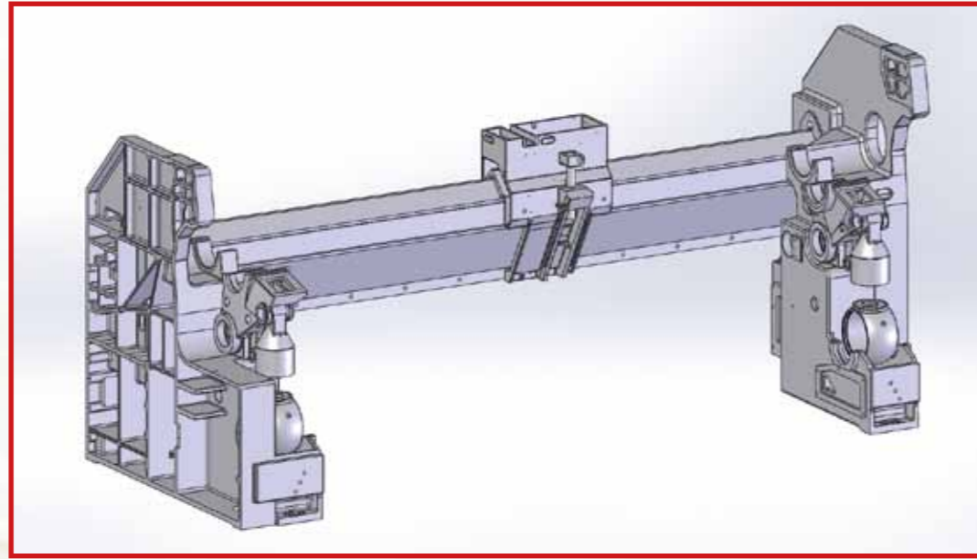
Struttura in ghisa. Iron cast structure.
