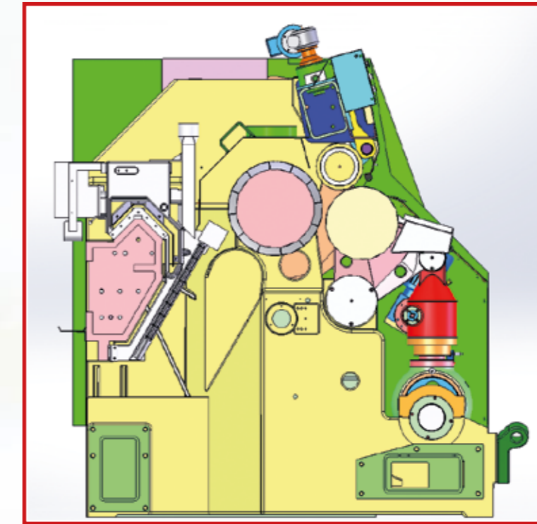
Sezione trasversale. Cross section.
